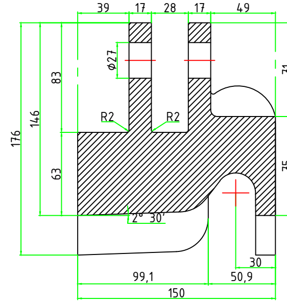
A-A Kesiti
